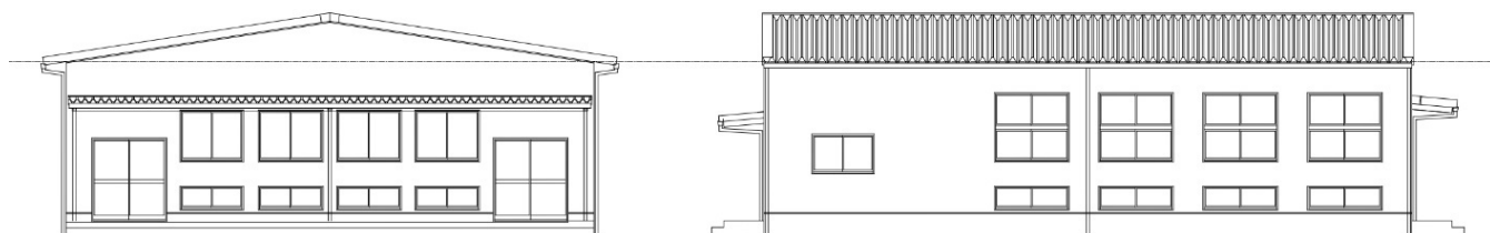
南立面図
